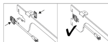
Posizionamento del connettore sul supporto mensola
