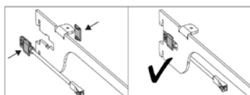
Posizionamento del connettore sul supporto mensola
